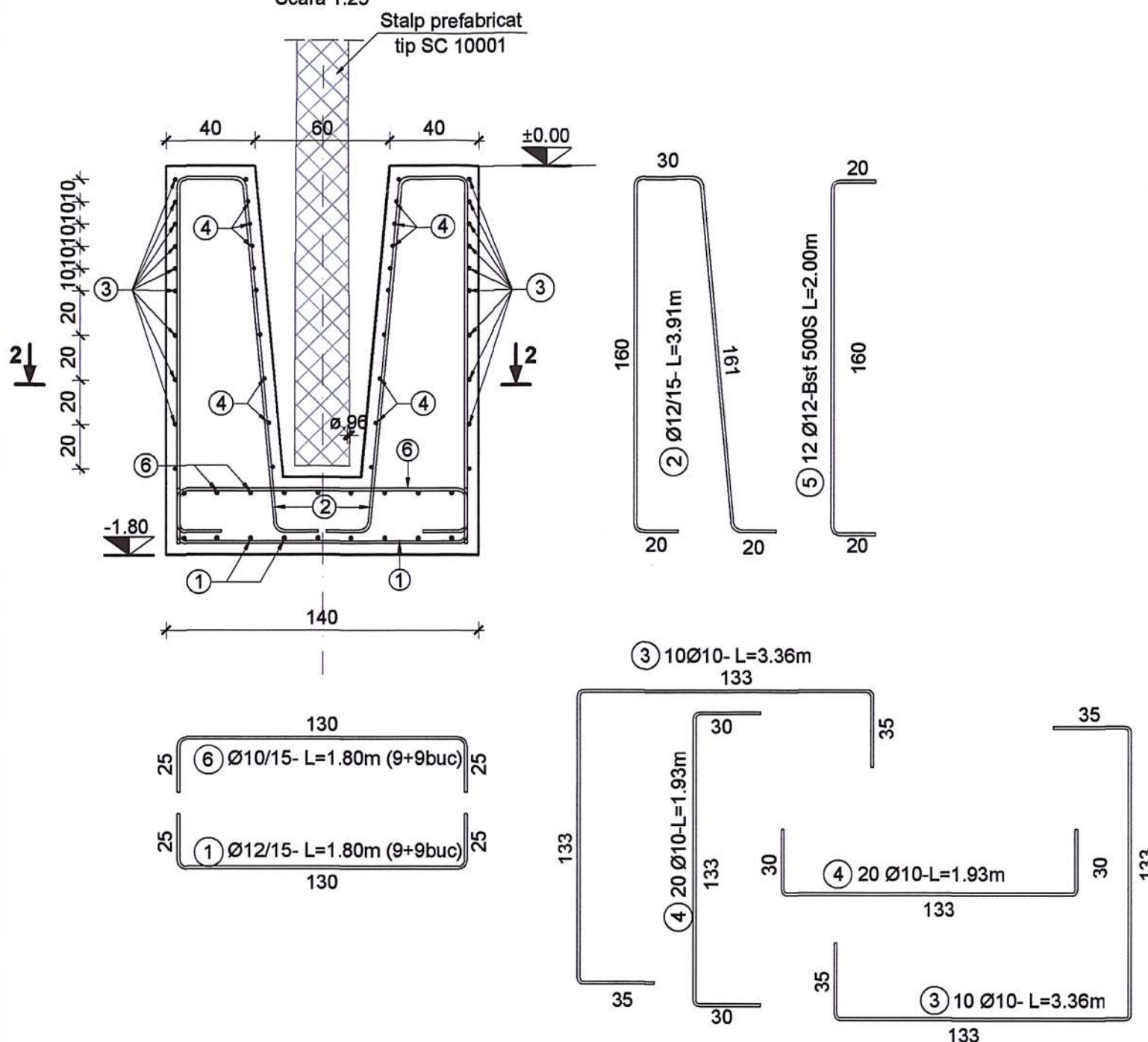
Sețiunea 1-1 Scara 1:25
