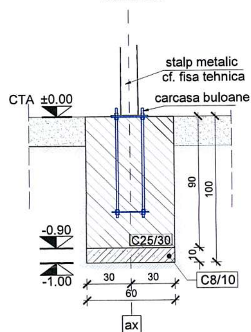
Detaliu fundatie stalp metalic iluminat Scara 1:25
