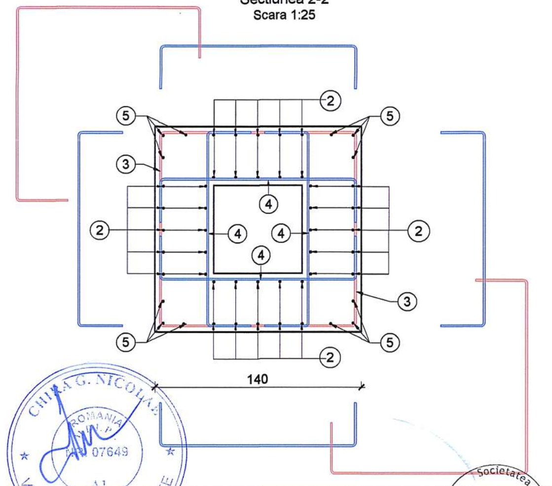
Sețiunea 2-2 Scara 1:25
