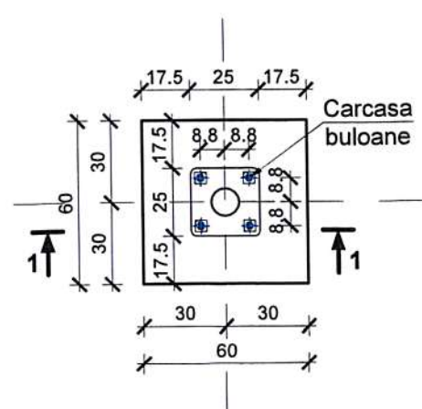
Fundatie stalp metalic iluminat Scara 1:25
