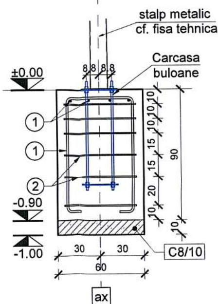
Sețiunea 1-1 Scara 1:25
