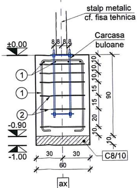
Sectiunea 1-1 Scara 1:25
